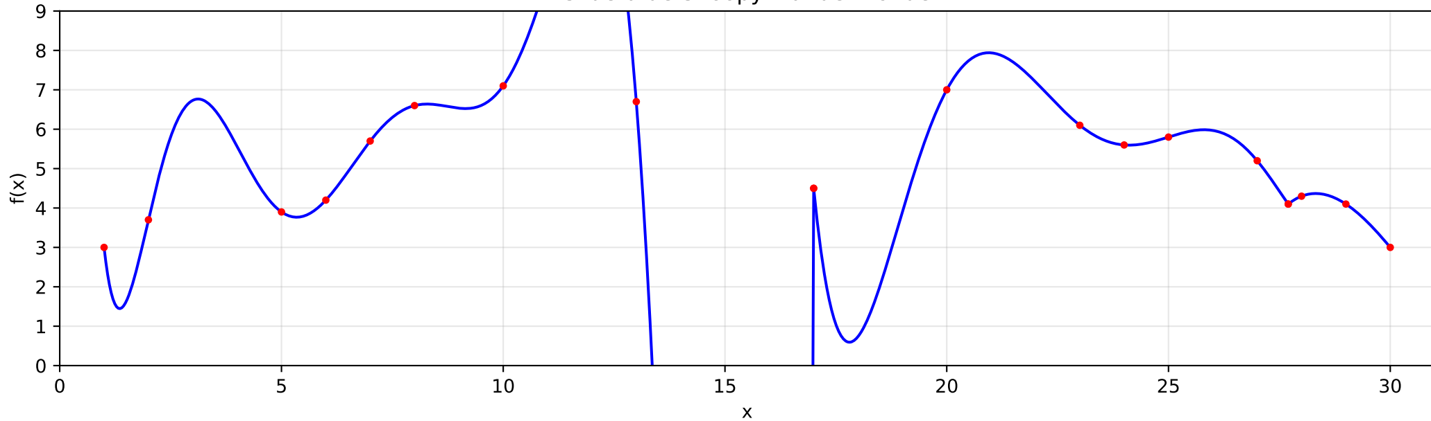
Silueta de Snoopy: Vandermonde
